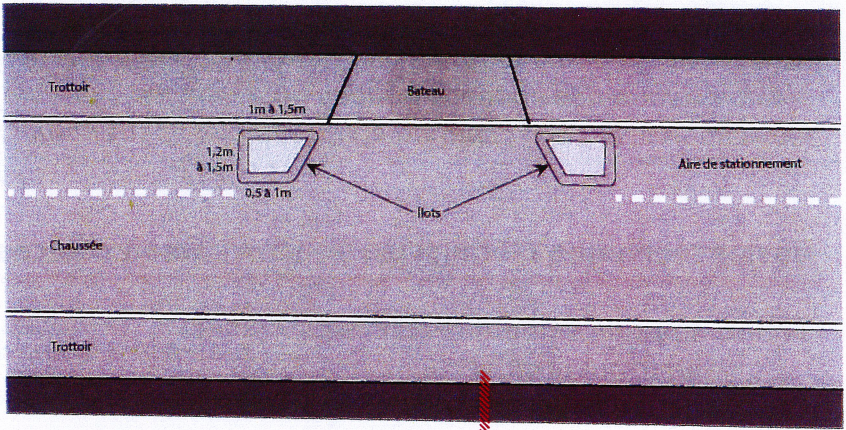
Vue en plan d'ilots de part et d'autre de l'entrée charretière / bateau
